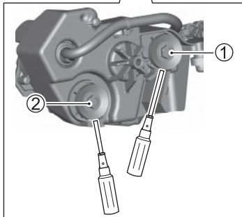
Feu de croisement
